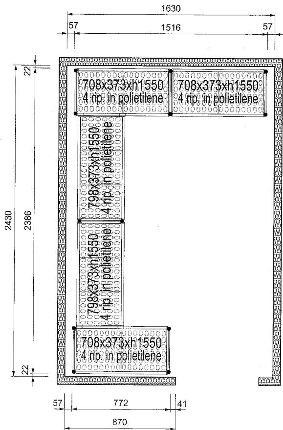
Boven aanzicht
